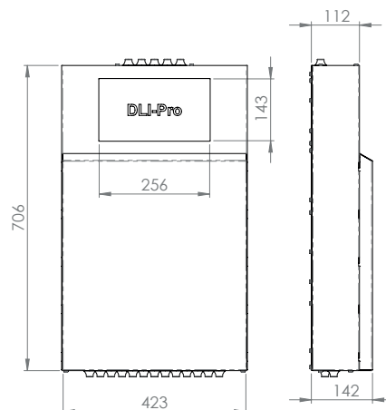
Maßzeichnung
